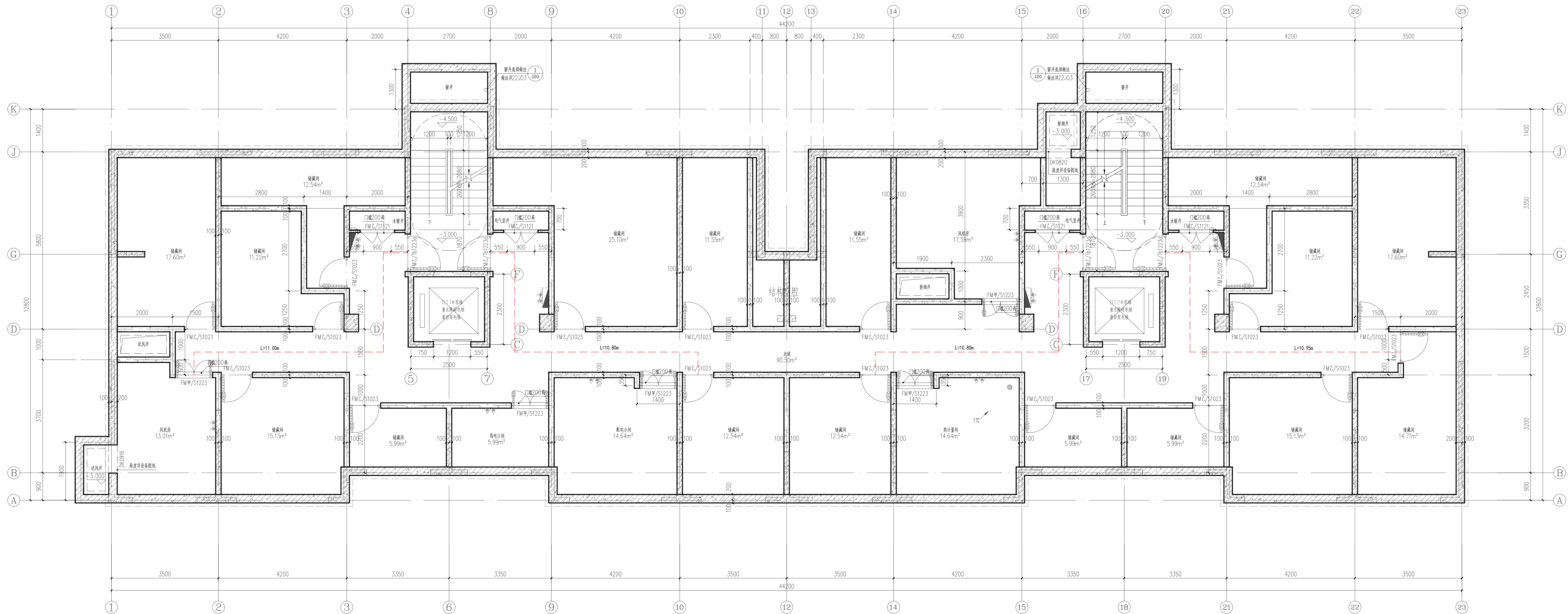
地下一层平面图 1:50
